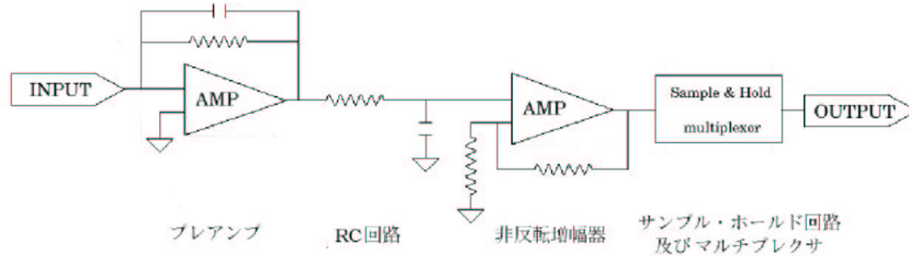
図 2.9: 回路の模式図
