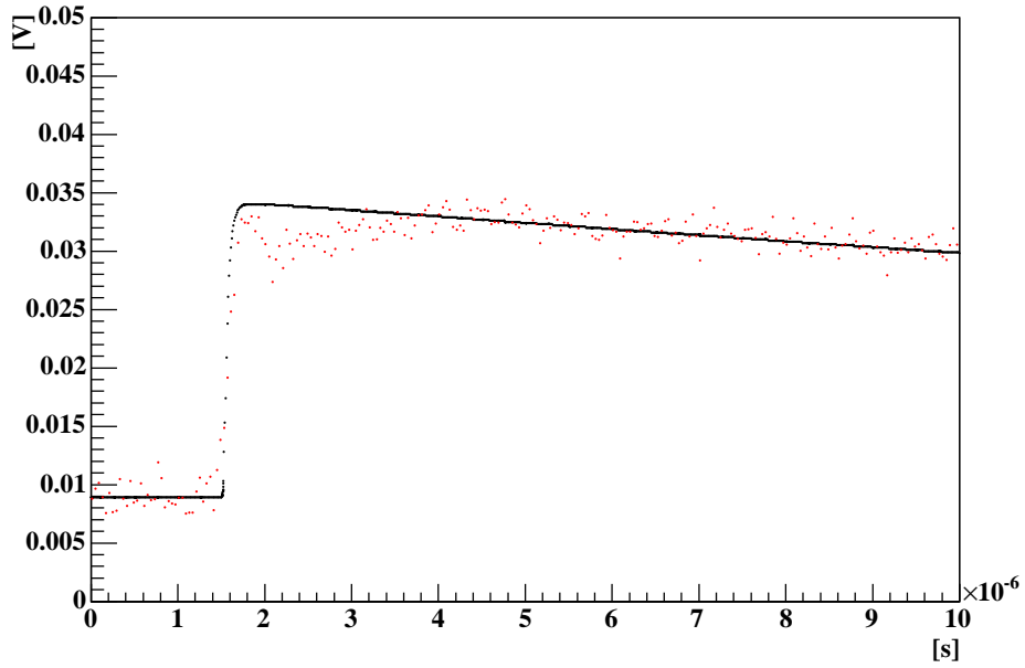
図 3.7: プレアンプにおけるシミュレーション及び実際の実出力波形
