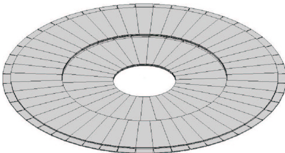
図 1.4: Pair Monitor(上が IP 側)
