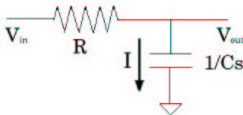
図 2.10: RC 回路
