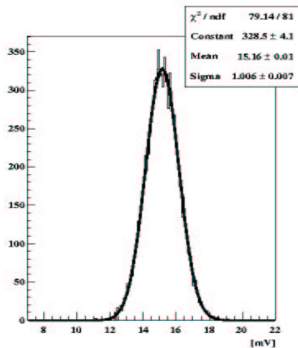
図 4.5: 再構成の波高の分布
