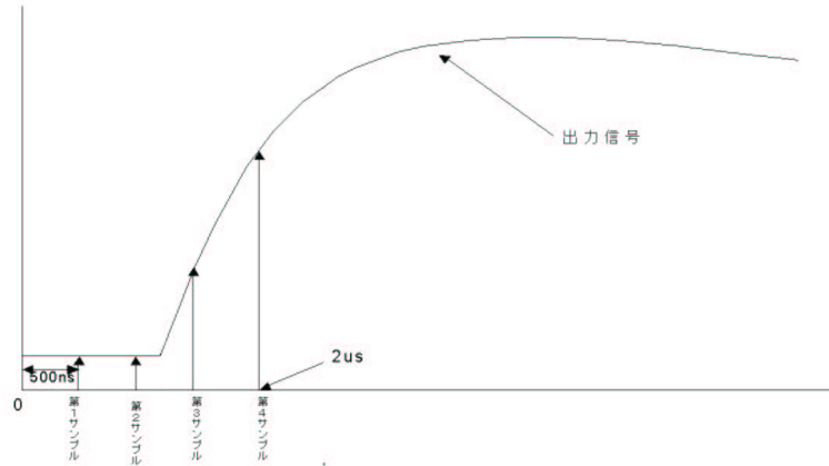
図 2.11: 波形の4点サンプル
